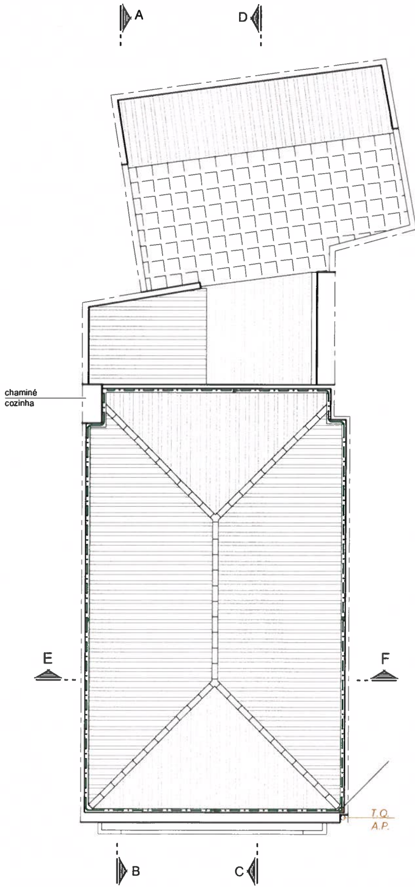
PLANTA DA COBERTURA
