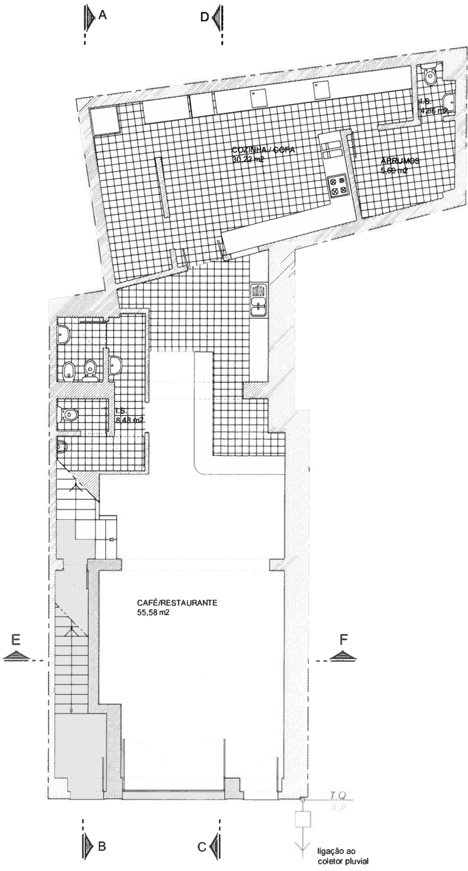
PLANTA DO R/CHÃO
