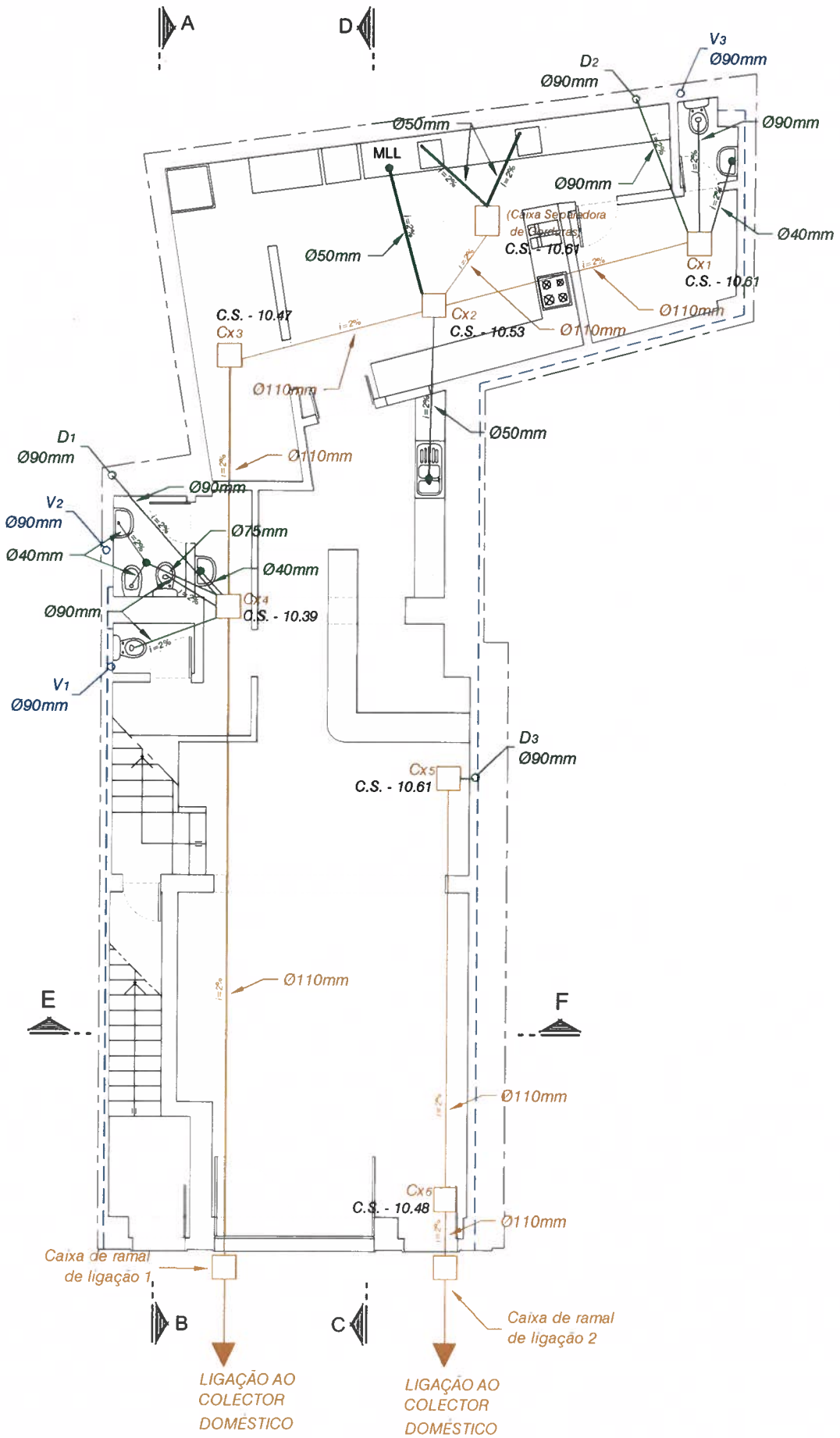
PLANTA DO R/CHÃO
