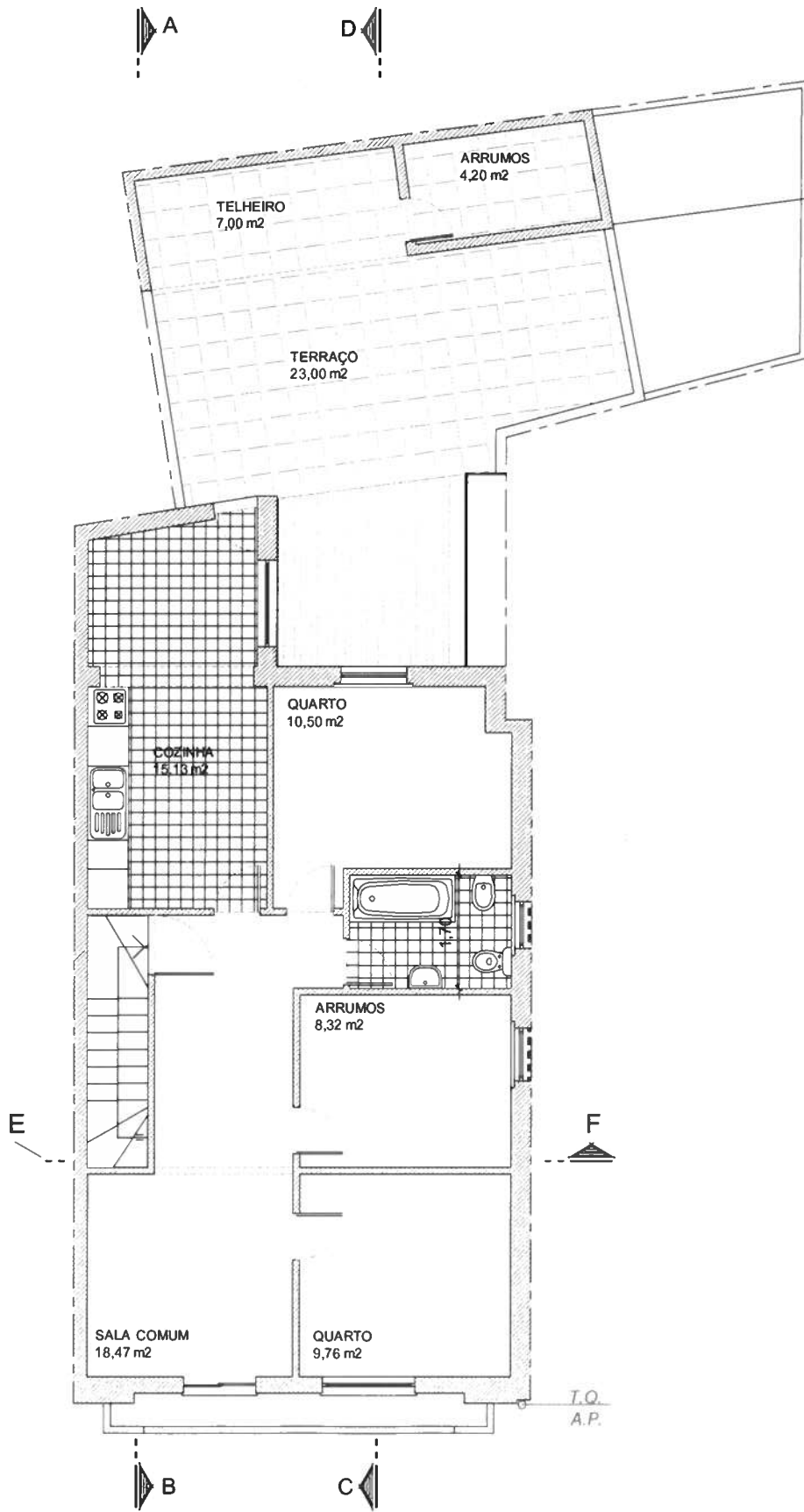
PLANTA DO 2º ANDAR
